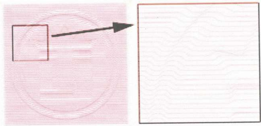
Gambar 8. Relief Motif
